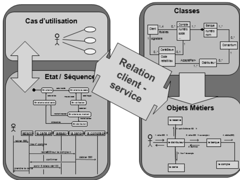
Figure 4. - Identification et granularité des services
